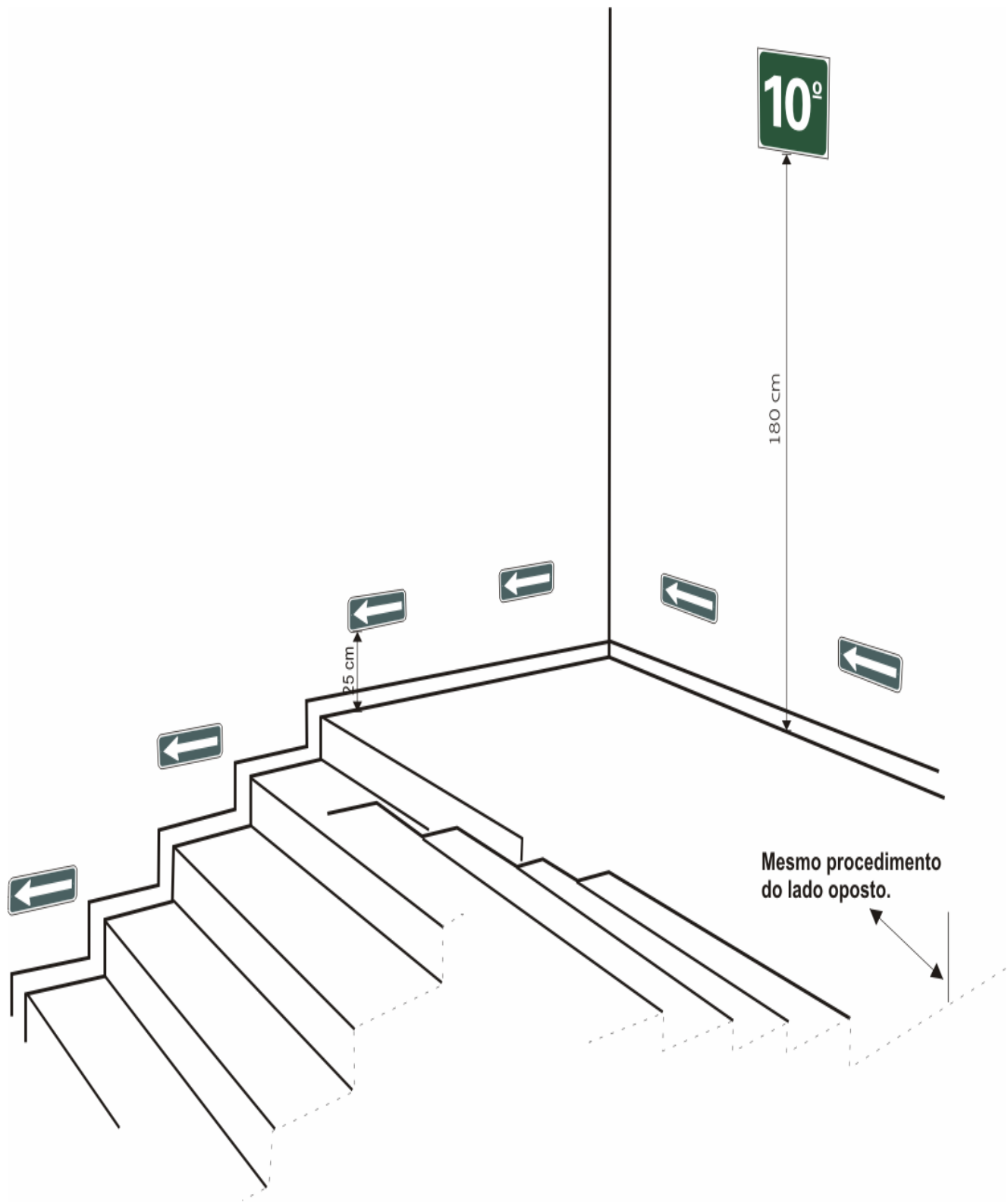
Figura 8 - Sinalização complementar. Exemplo de rodapé
