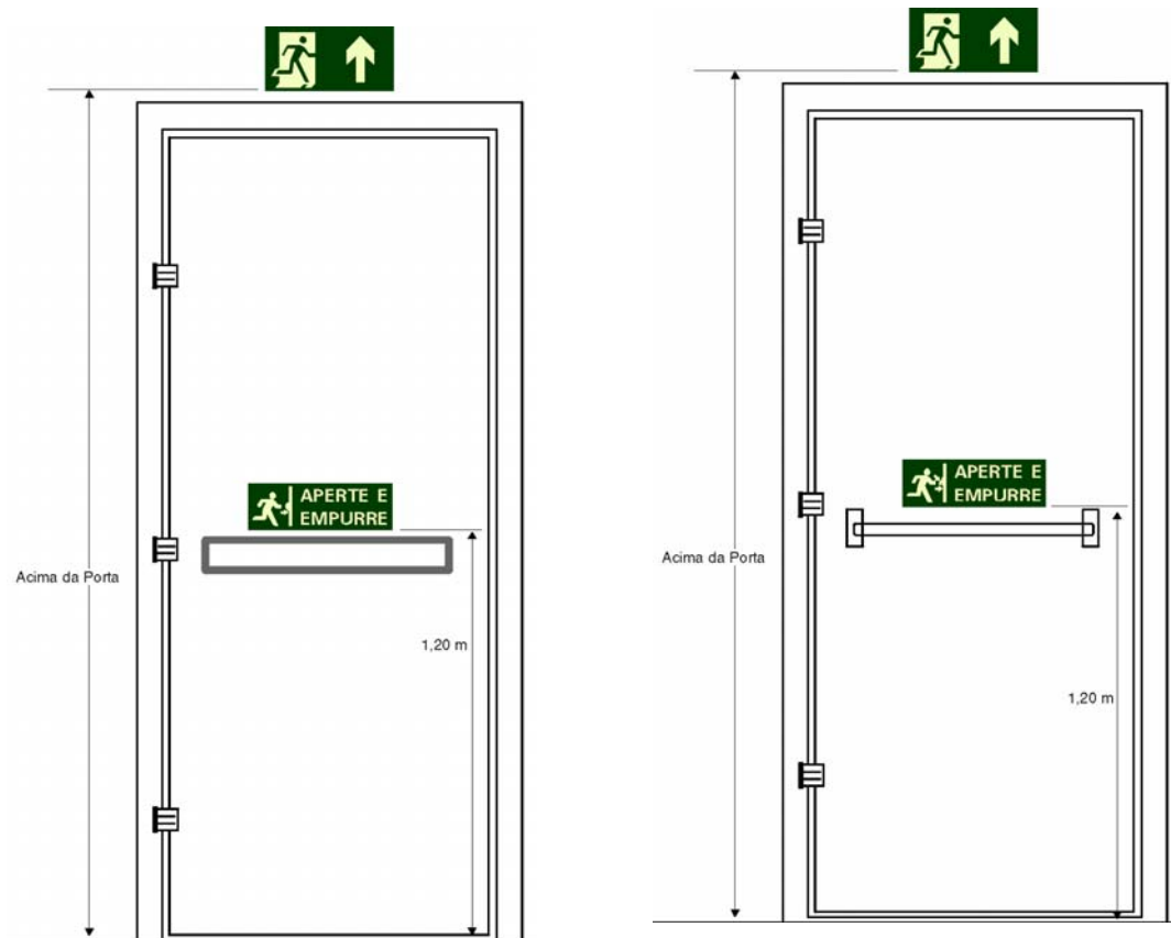
Figura 5 – Sinalização de portas com barras antipânico (modelos 1 e 2)
