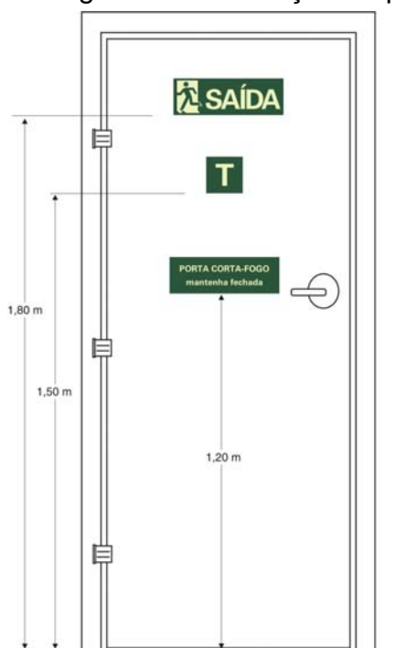
Figura 2 - Sinalização de porta corta-fogo (vista do hall )
